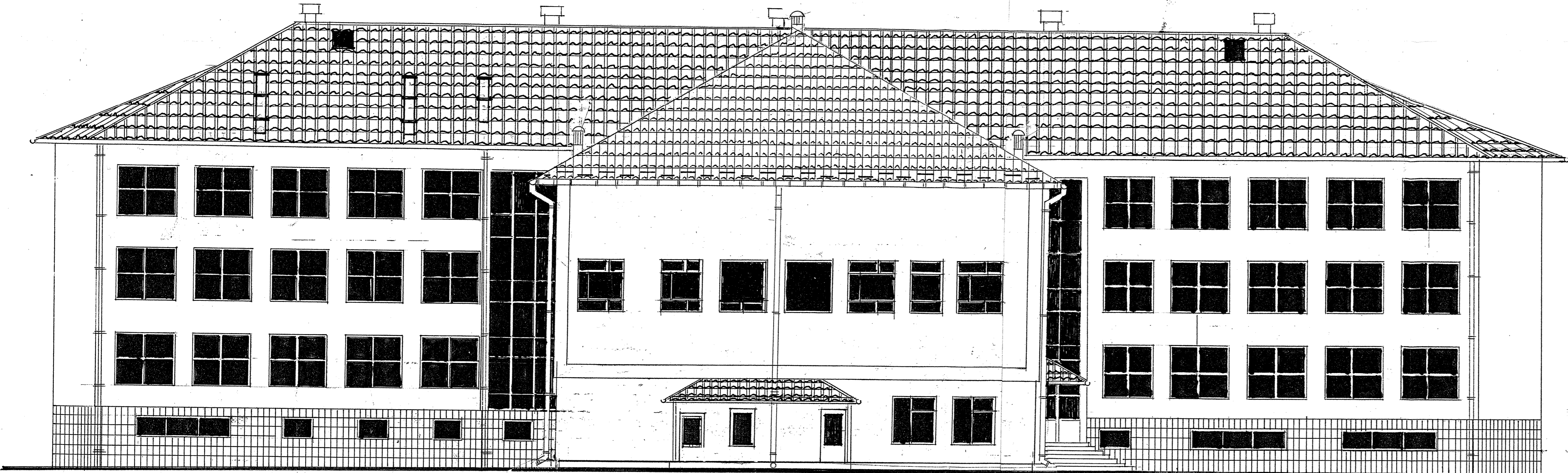
ELEWACJA ZACHODNIA 1:100
